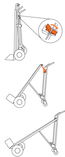
CONVERSIÓN DE 2 RUEDAS A ASISTIDO
