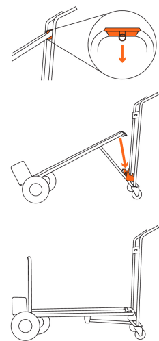
CONVERSIÓN DE ASISTIDO A 4 RUEDAS
