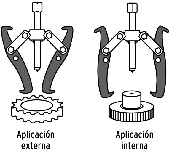
Quijadas ajustables reversibles
